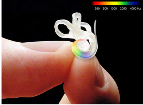
ན་བའི་དྲུང་འབྲིལ། Cochlea
